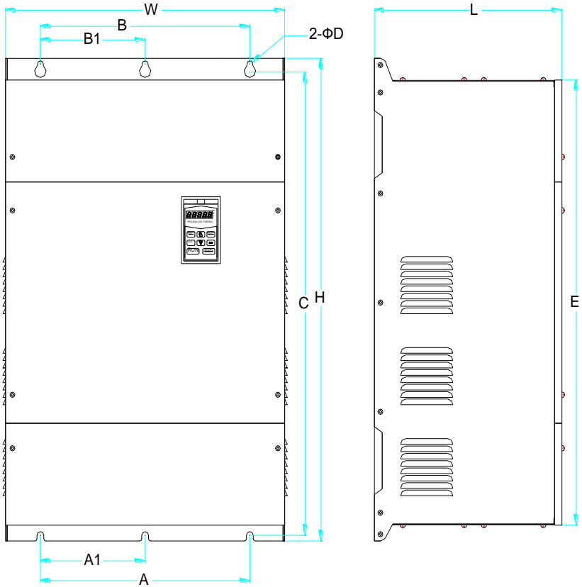
图 2-7: 壁挂式安装 (55KW-450KW)
