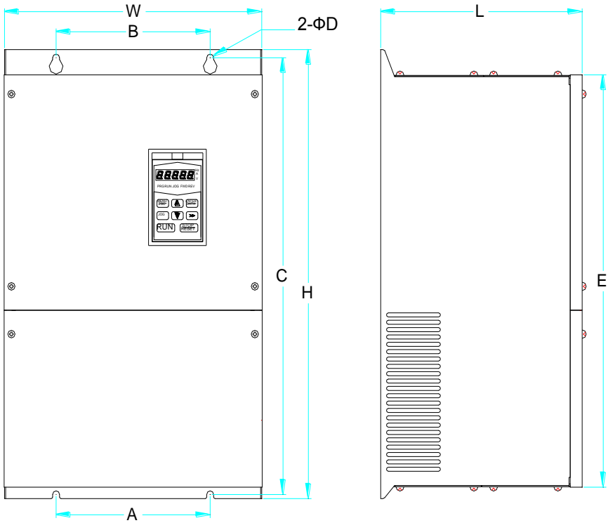
图 2-6: 壁挂式安装 (22KW-45KW)
