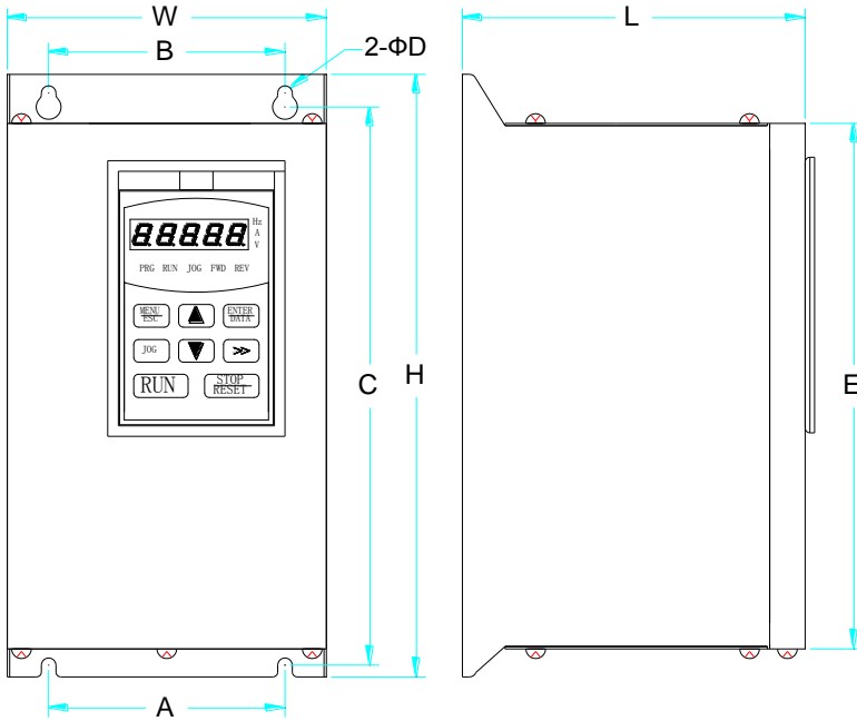
图 2-5: 壁挂式安装 (5.5KW-18.5KW)
