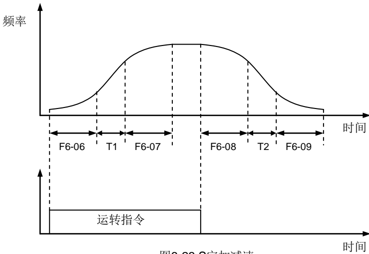
图6-23 S字加减速
