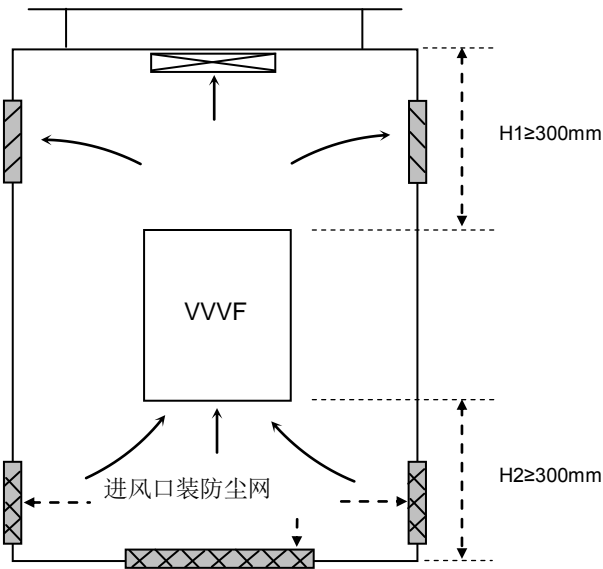
附图 1-1 多粉尘现场 变频器安装示意图
