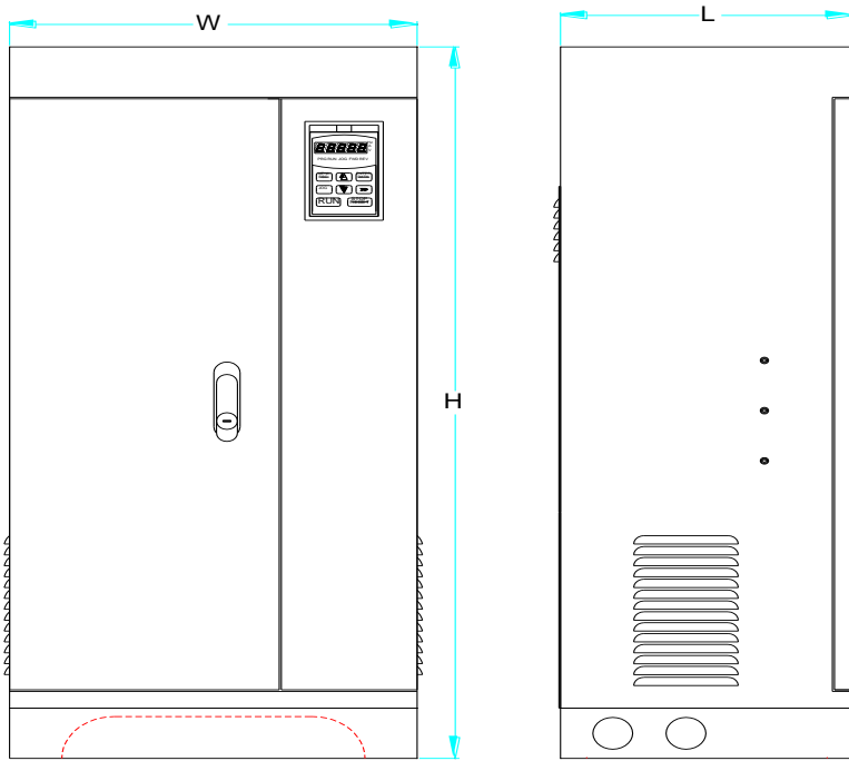
图 2-8: 落地式安装 (11KW-1000KW)
