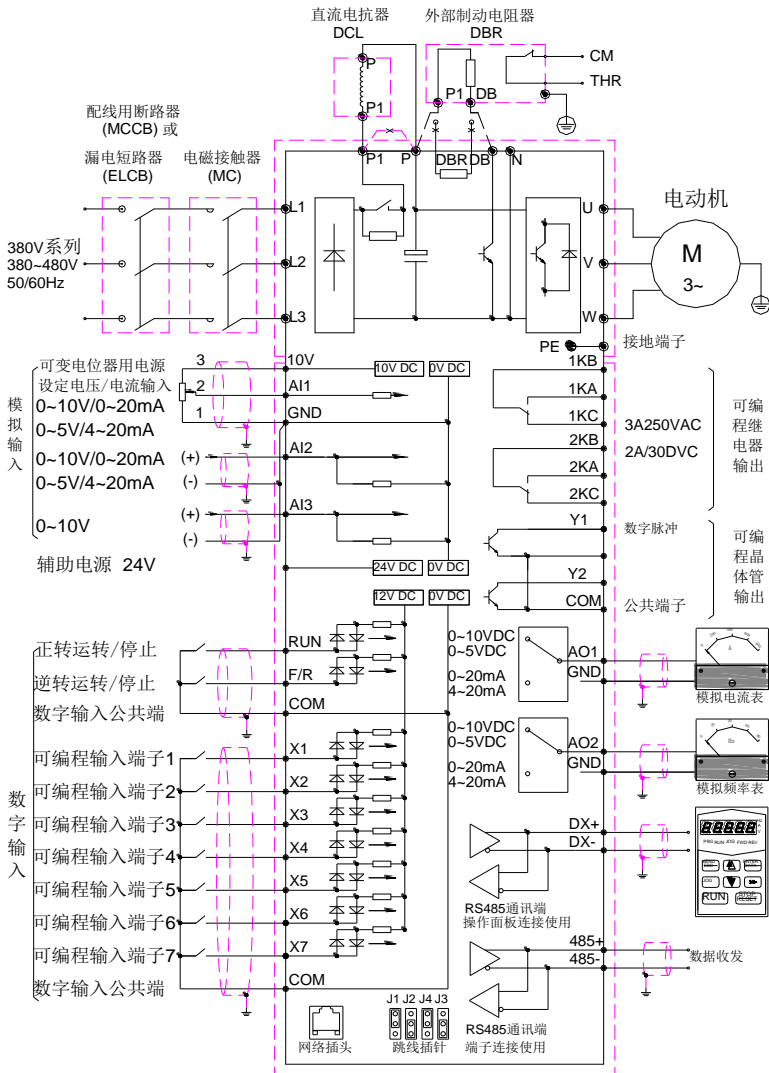
变频器接线图
