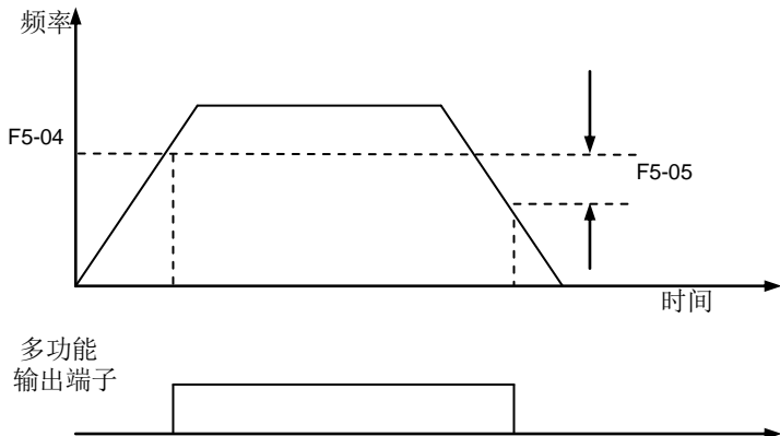
图 6-11 任意检出频率 1
