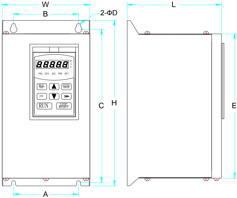
图 1：壁挂式安装（0.75KW-15KW）
