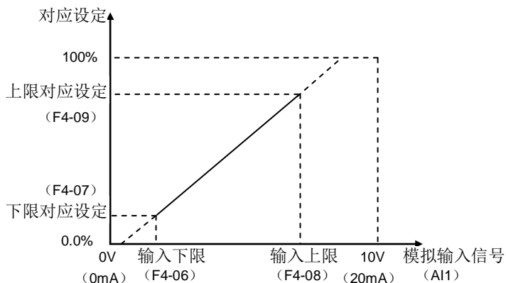
图 6-7 模拟输入上下限示意图
