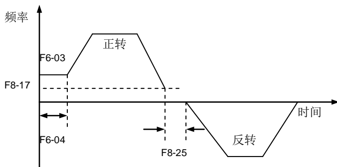
图 6-31 正反转死区时间
