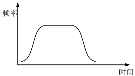
图 6-22 曲线加减速
