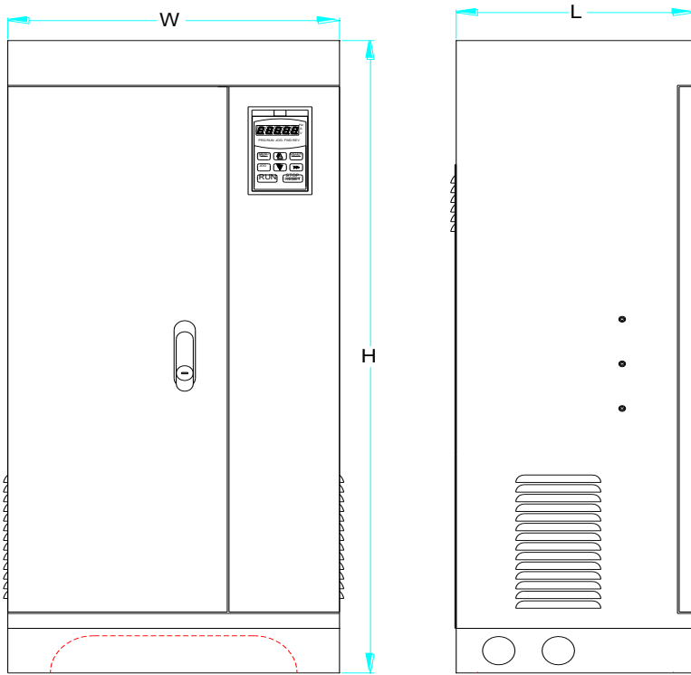
图 4：落地式安装（7.5KW-800KW）
