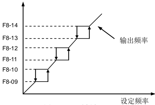
图 6-29 回避频率
