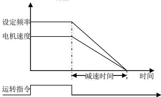
图 6-24 减速停车
