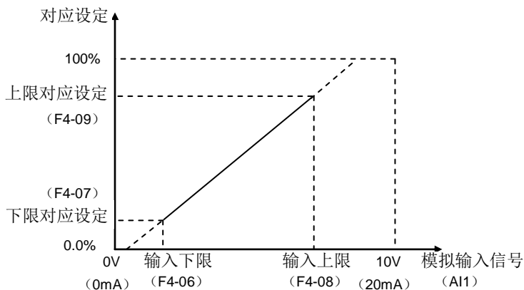
图 6-7 模拟输入上下限示意图
