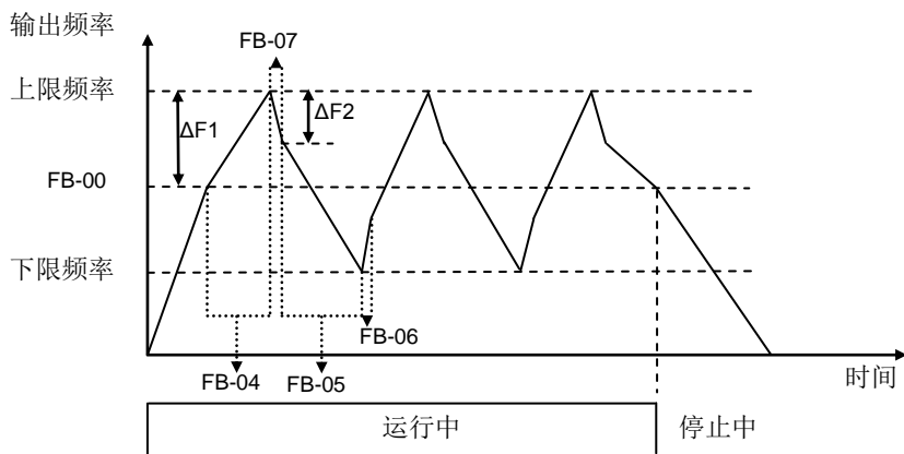
图 42 摆频范围和加减速
