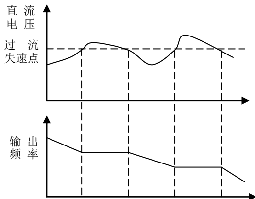
图 6-33 过压失速
