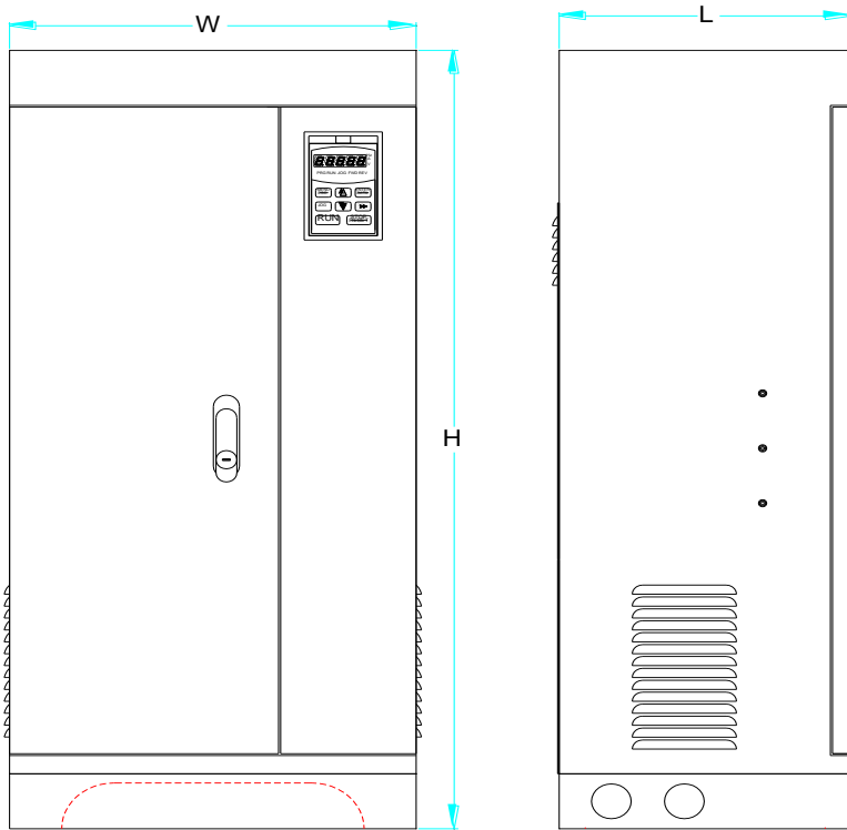
图 4: 落地式安装 (11KW-1000KW)
