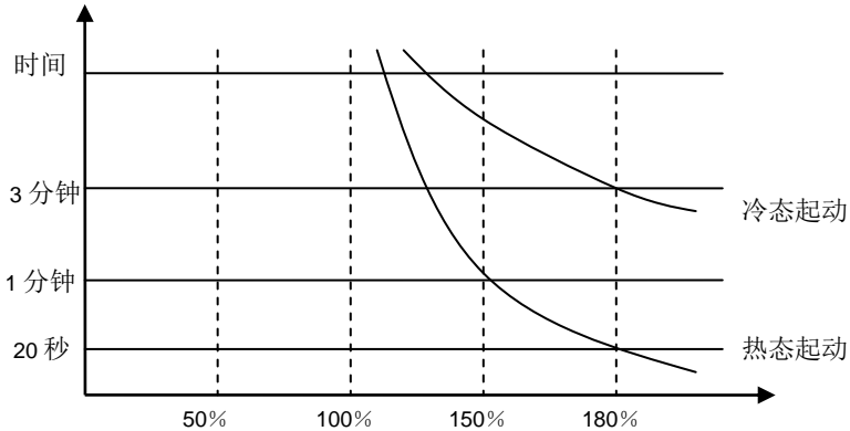
图 6-32 电子热保护
