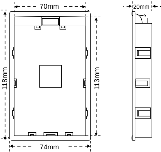
图 2-4 键盘托盘尺寸
