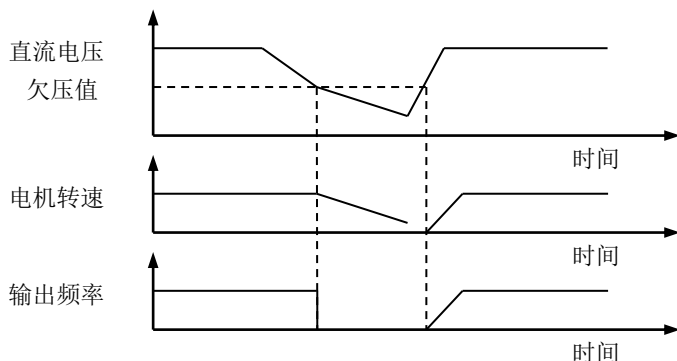
图 6-17 电恢复时频率从零起动
