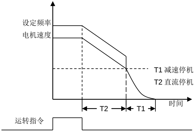
图 6-26 减速停车加直流制动
