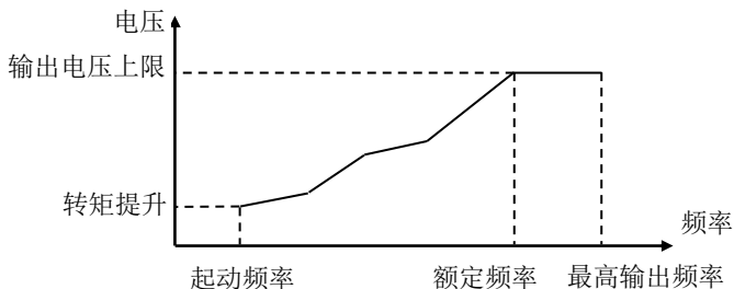
任意 V/F 曲线
