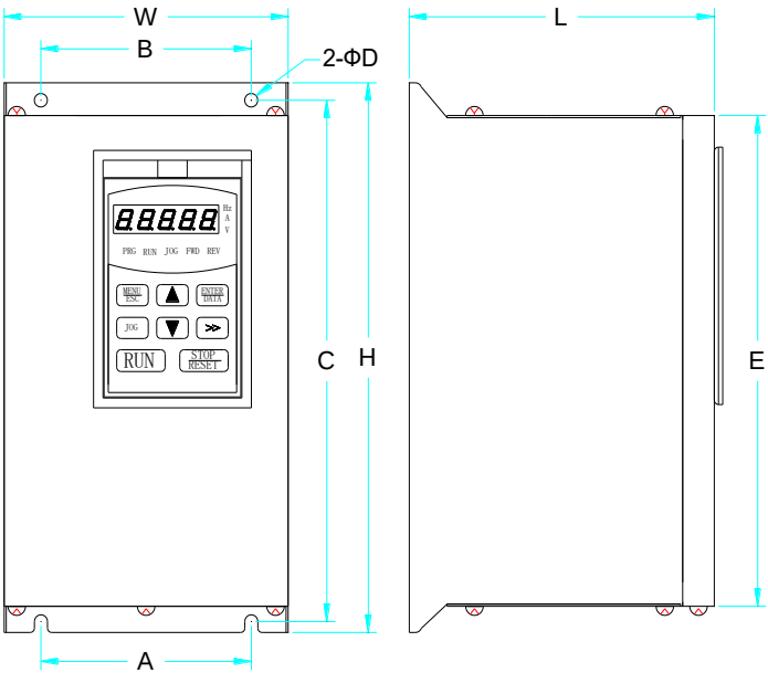
图 1：壁挂式安装（1.5KW-18.5KW）
