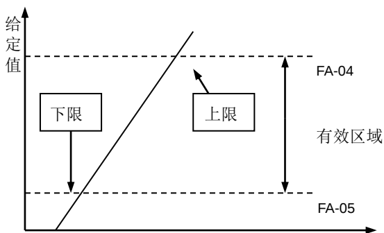
图 6-38 给定值限制
