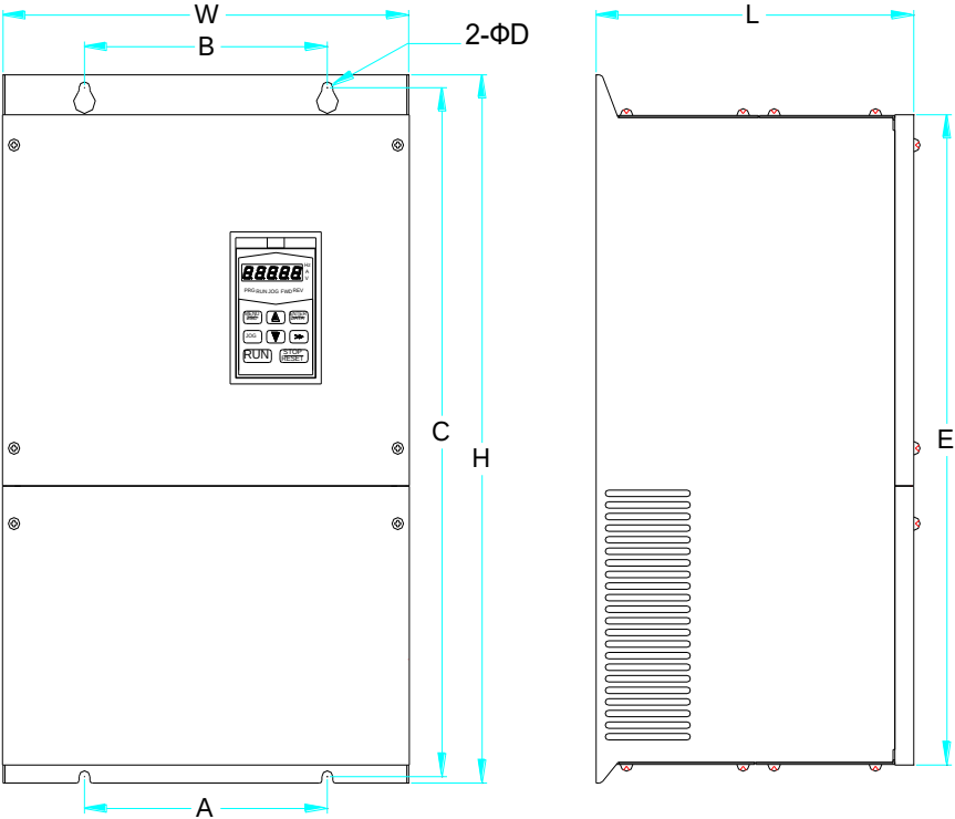
图 2：壁挂式安装（18.5KW-45KW）
