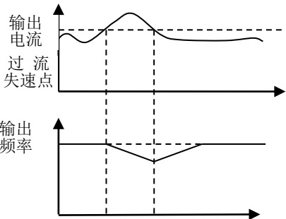
图 6-35 恒速运行中过流失速控制
