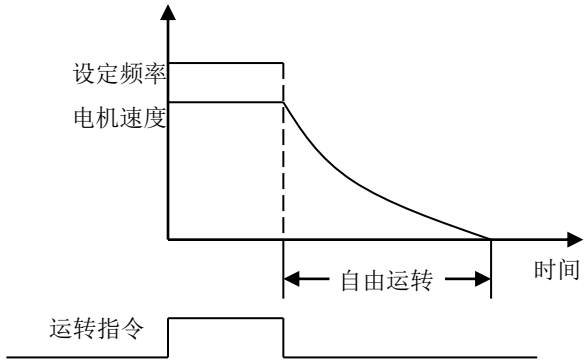
图 6-25 自由停车
