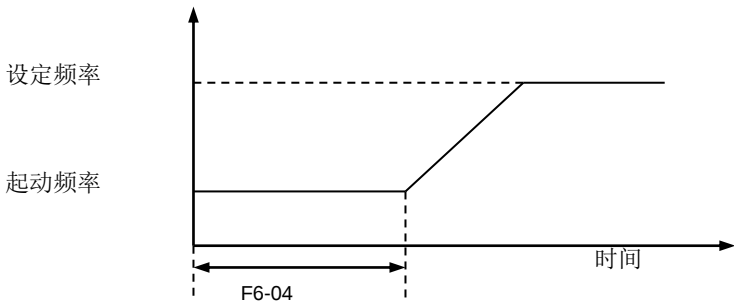
图 6-20 起动频率持续时间
