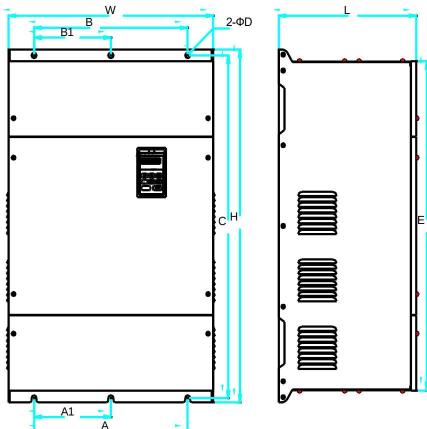
图 3：壁挂式安装（55KW-400KW）
