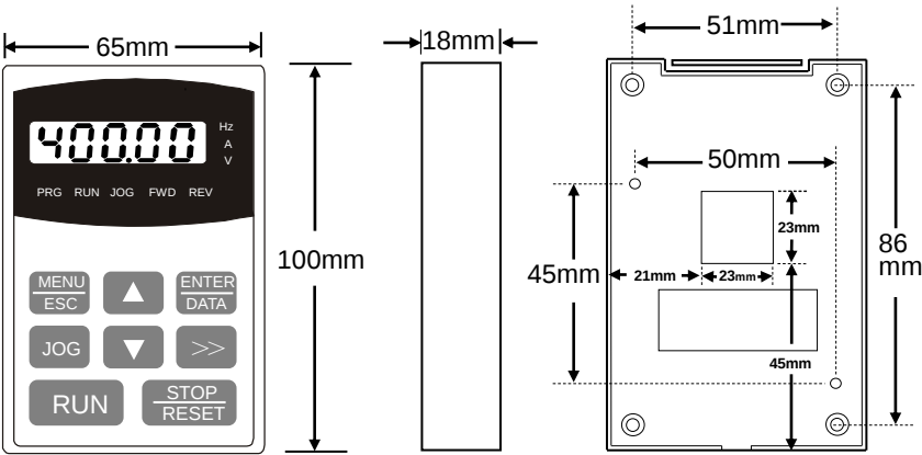
图 2-3 操作键盘尺寸
