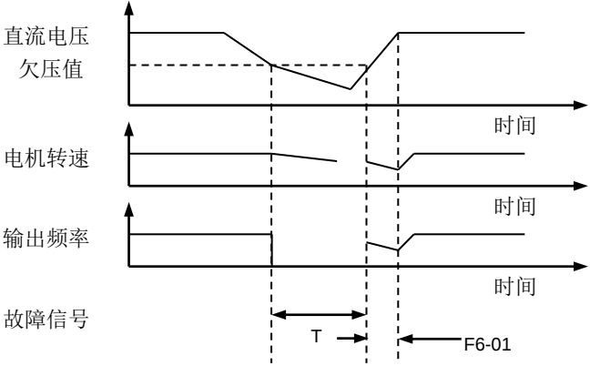
图 6-19 跟踪起动 T < F6-02
