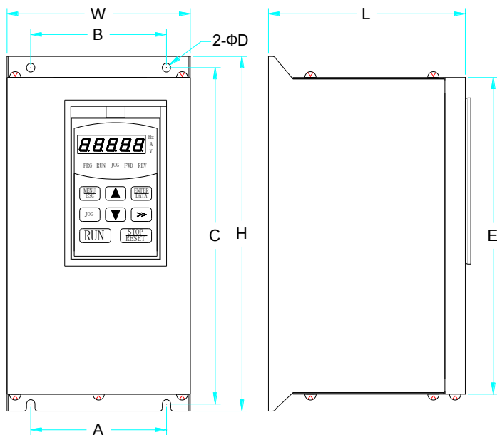
图 1：壁挂式安装（0.75KW-15KW）
