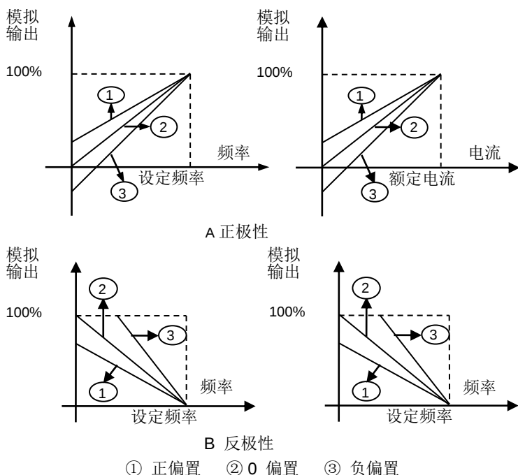
图 6-14 模拟输出信号示意图
