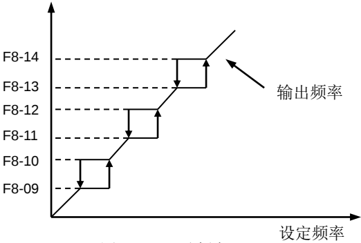
图 6-29 回避频率
