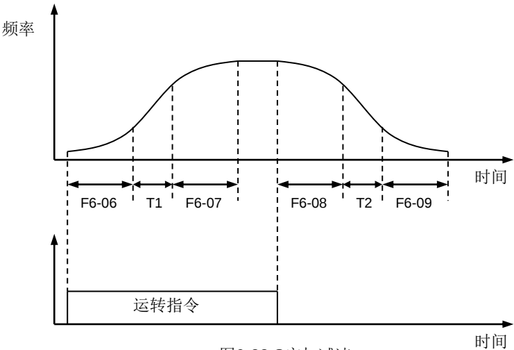
图6-23 S字加减速
