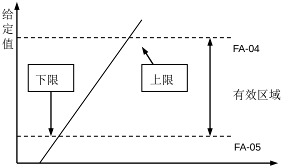
图 6-37 给定值限制
