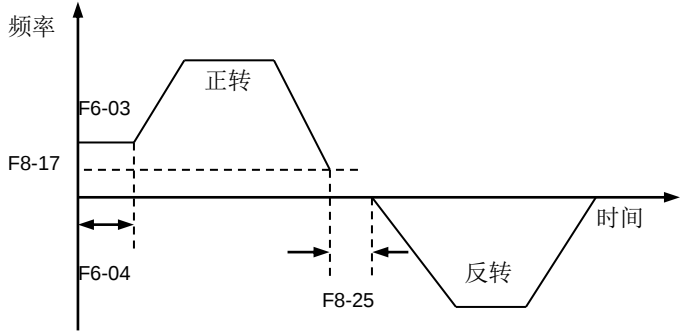
图 6-30 正反转死区时间
