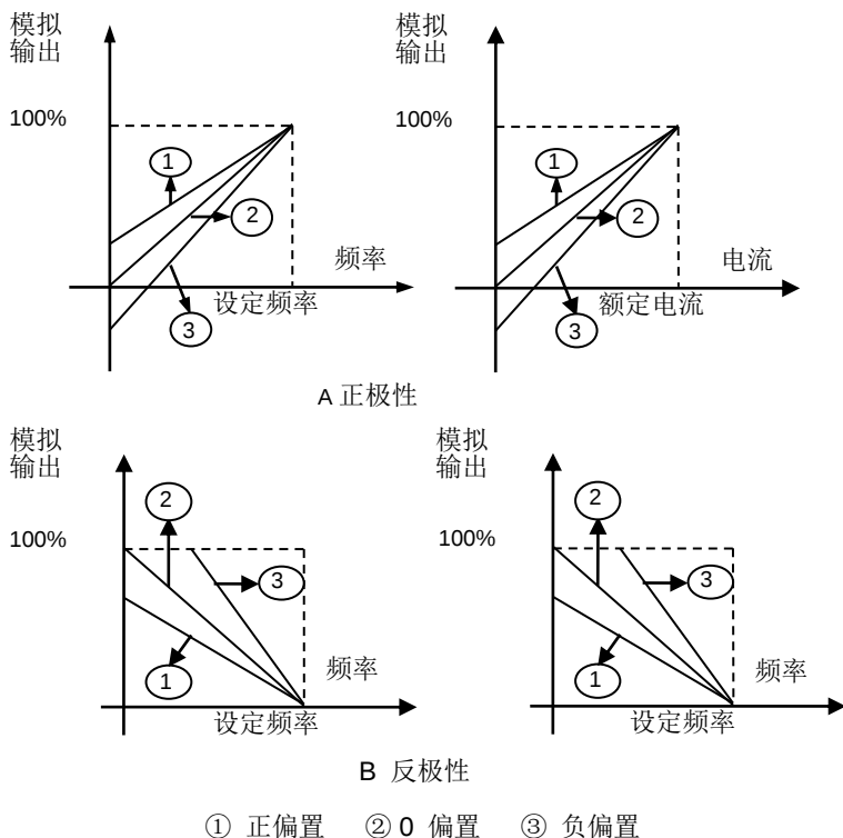
图 6-13 模拟输出信号
