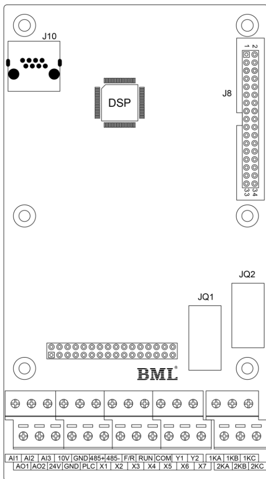
图 3-4 主板示意图
