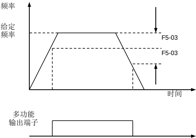
图 6-10 频率到达宽度
