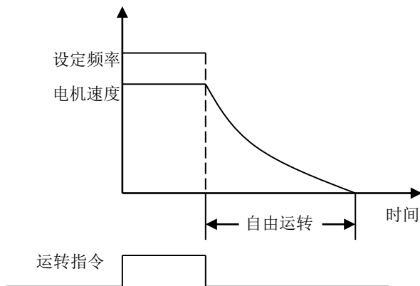
图 6-24 自由停车
