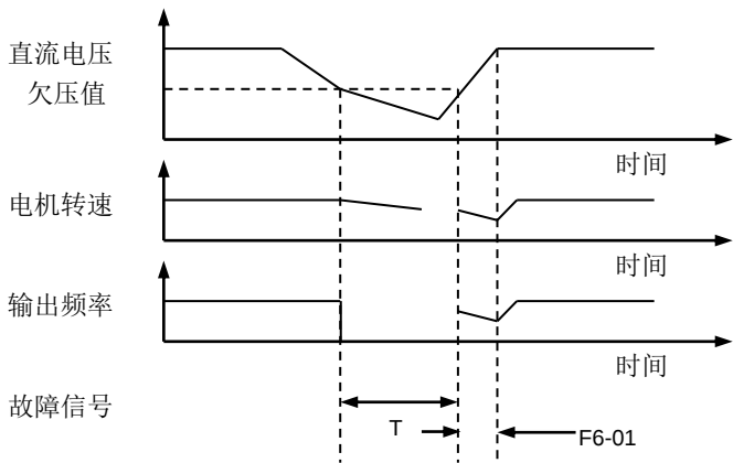
图 6-18 跟踪起动 T < F6-02
