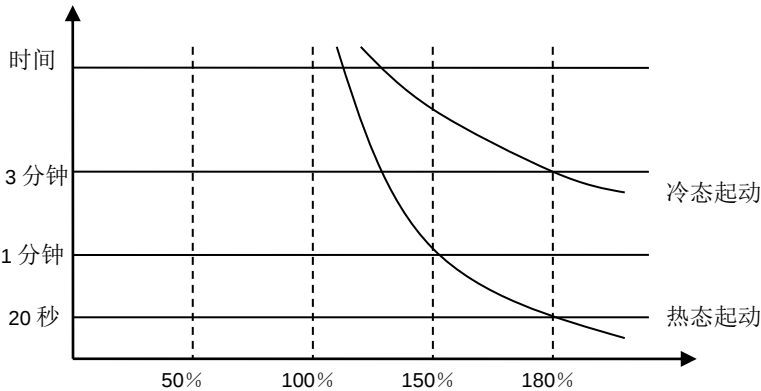
图 6-31 电子热保护
