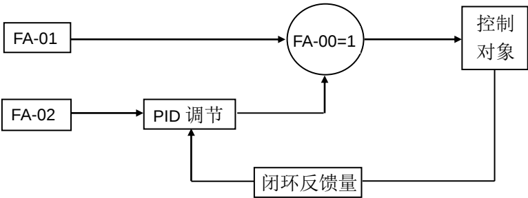
图 6-36 开环给定+PID 运行
