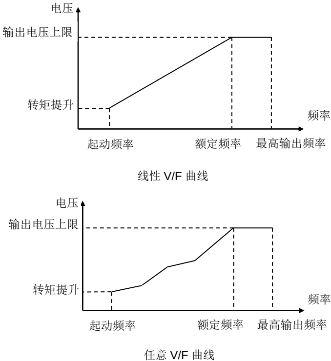
图 6-3：V/F 曲线图
