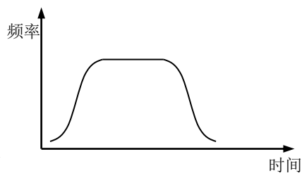
图 6-21 曲线加减速
