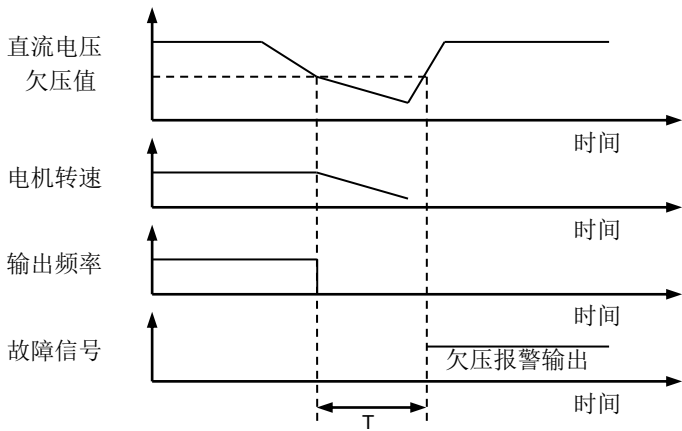
图 6-17 停电超时欠压保护 T > F6-02
