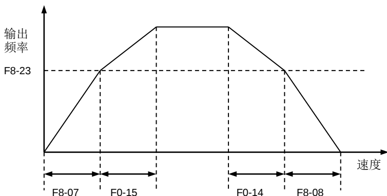
图 6-29 加减速切换频率
