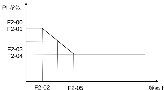
图 6-2: PI 参数示意图
