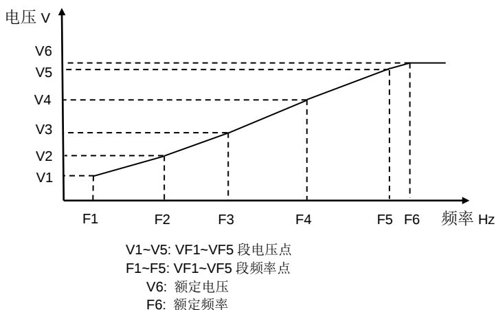
图 6-4 自定义 V/F 曲线图
