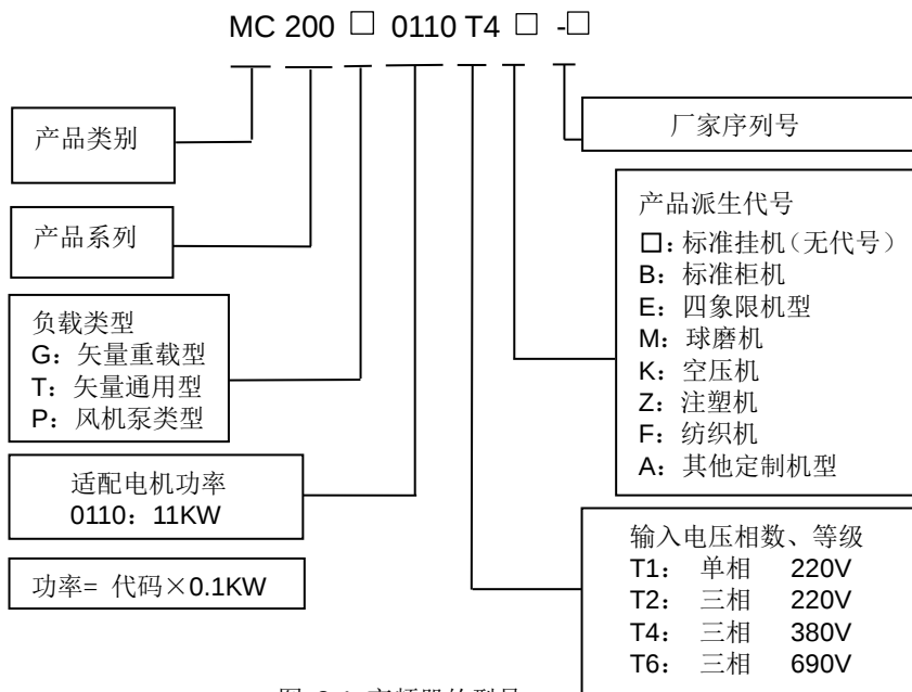
图 2-1 变频器的型号
