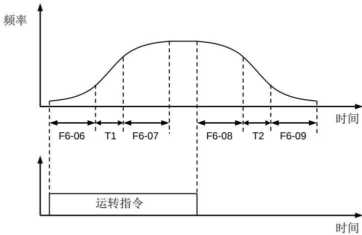
图6-22S字加减速
