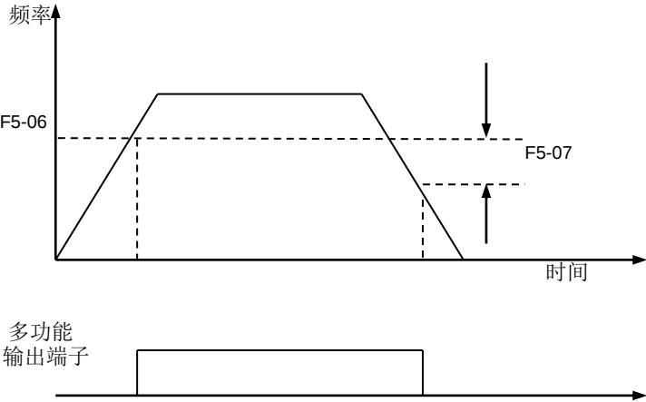
图 6-12 任意检出频率 2
