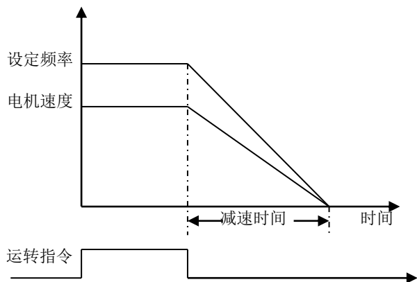
图 6-23 减速停车
