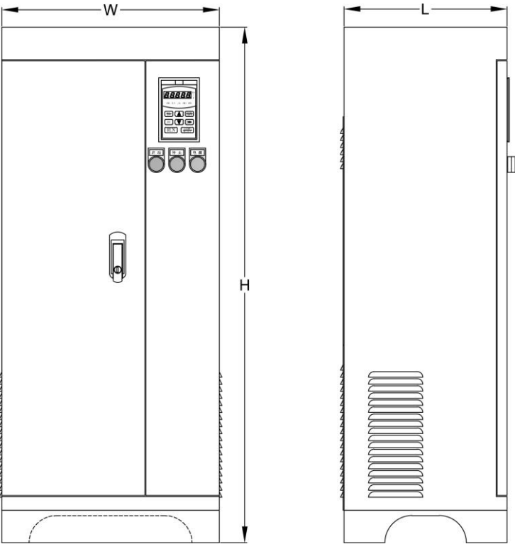
图 4：落地式安装（11KW-1000KW）
