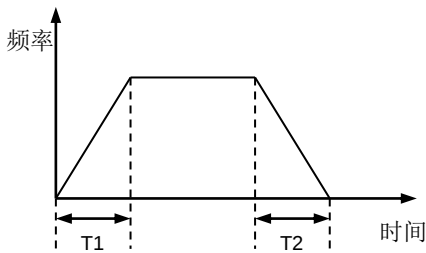
图 6-20 直线加减速
