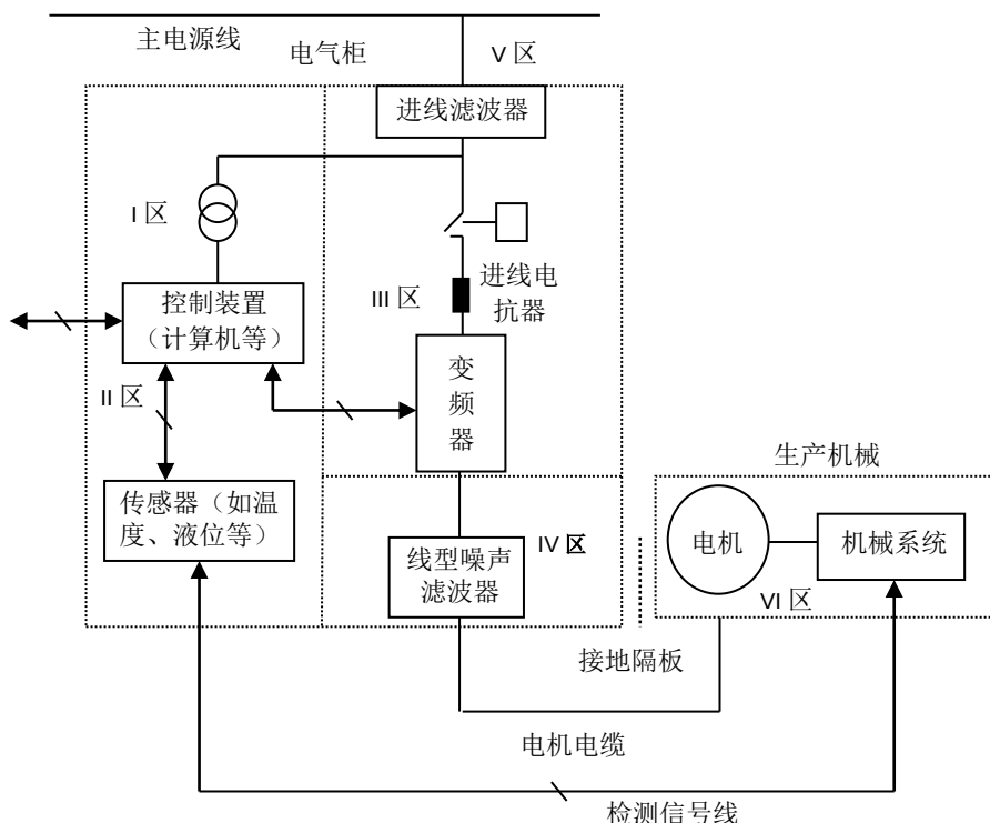
附图 2-8 变频器 EMC 安装区域划分示意图
