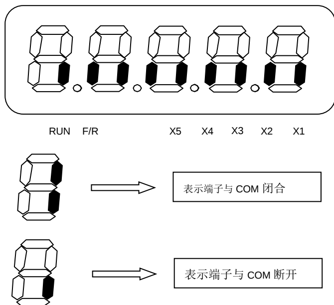
图 6-26 输入端子状态显示
