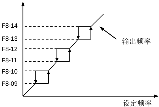
图 6-28 回避频率
