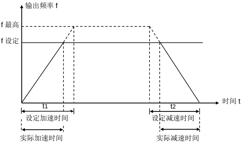
图 6-1：加减速时间示意图
