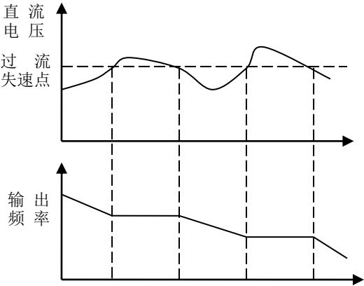
图 6-32 过压失速
