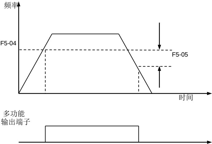
图 6-11 任意检出频率 1
