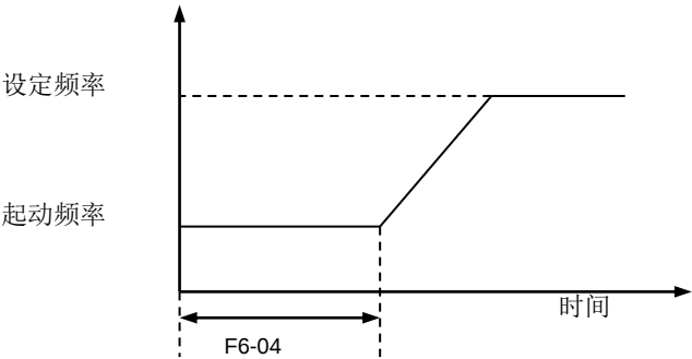
图 6-19 起动频率持续时间
