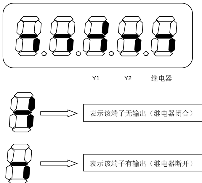
图 6-27 输出端子状态显示
