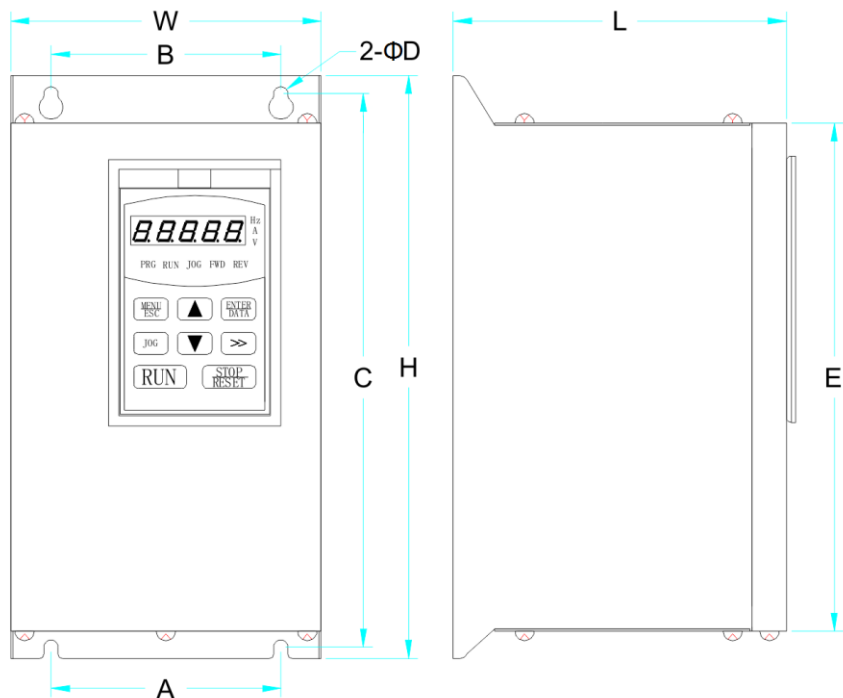
图 1：壁挂式安装（1.5KW-22KW）
