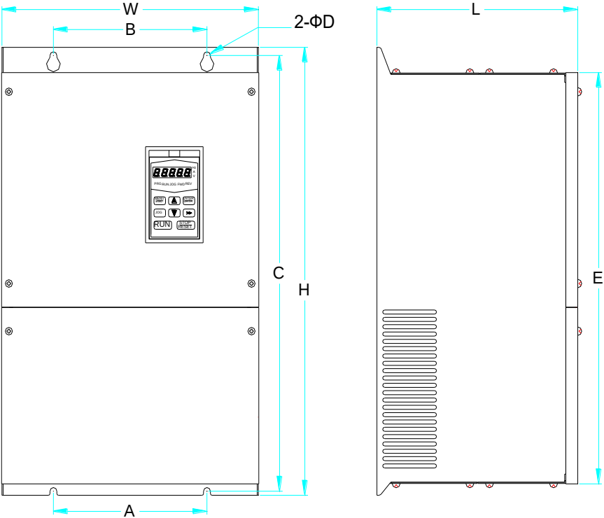
图 2：壁挂式安装（30KW-55KW）
