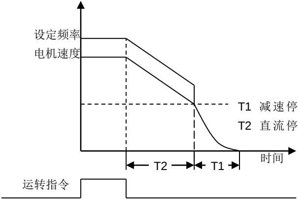
图 6-25 减速停车加直流制动
