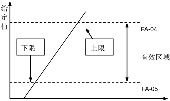
图 6-37 给定值限制
