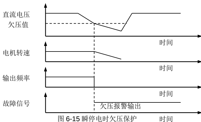
图 6-15 瞬停电时欠压保护
