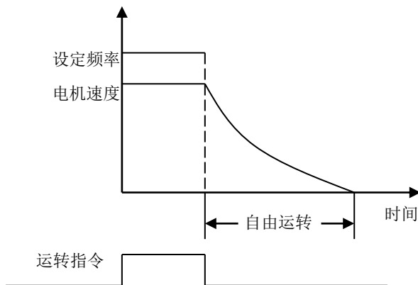
图 6-24 自由停车
