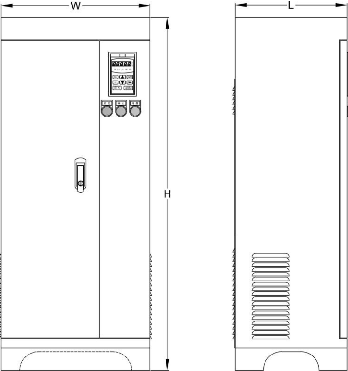
图 4：落地式安装（11KW-1000KW）
