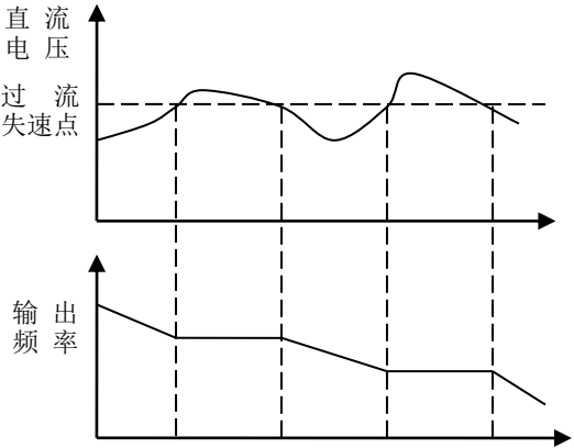
图 6-32 过压失速
