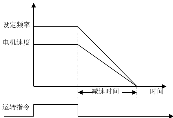
图 6-23 减速停车
