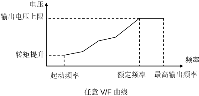
图 6-3：V/F 曲线图
