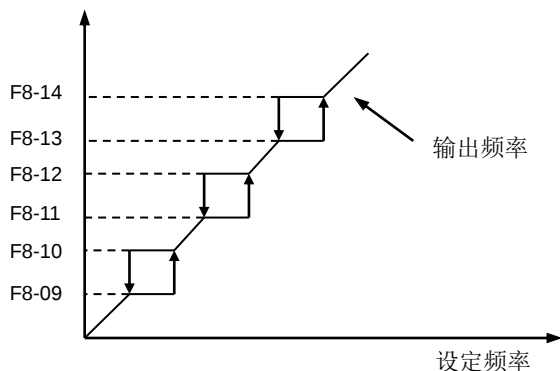
图 6-28 回避频率
