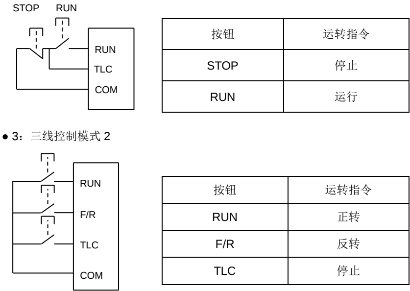
图 6-6 外控端子控制运行方式示意图
