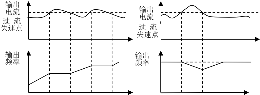
图 6-33 加速运行中过流失速控制
