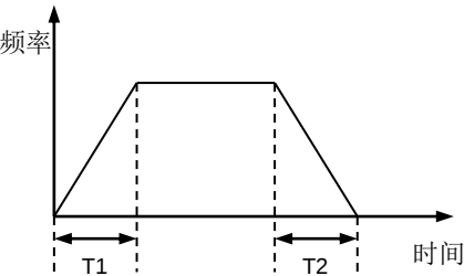
图 6-20 直线加减速
