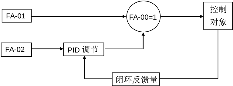
图 6-36 开环给定+PID 运行
