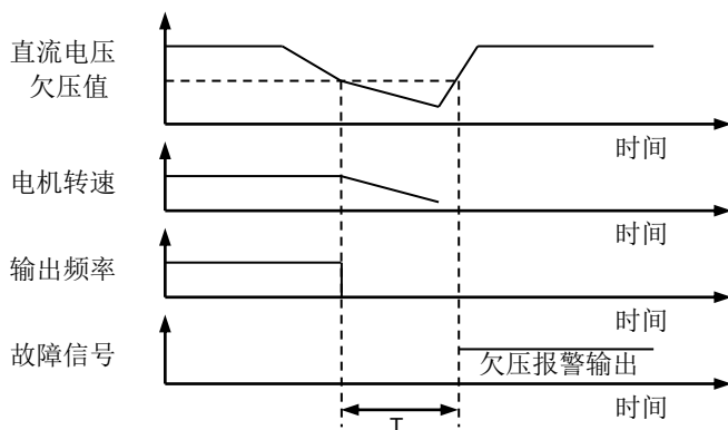
图 6-17 停电超时欠压保护 T > F6-02
