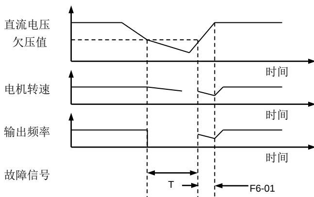
图 6-18 跟踪起动 T < F6-02
