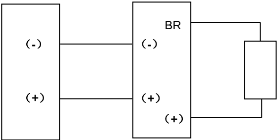
变频器 制动单元 制动电阻
