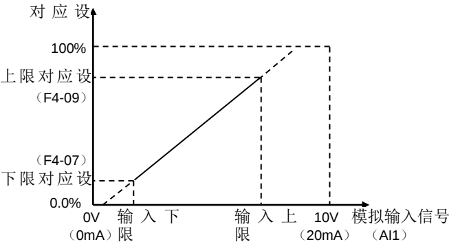
图 6-7 模拟输入上下限示意图
