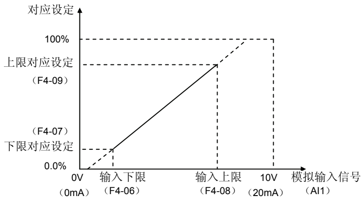
图 6-7 模拟输入上下限示意图
