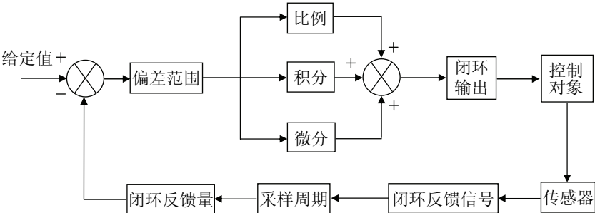
图 6-36 单一 PID 运行
