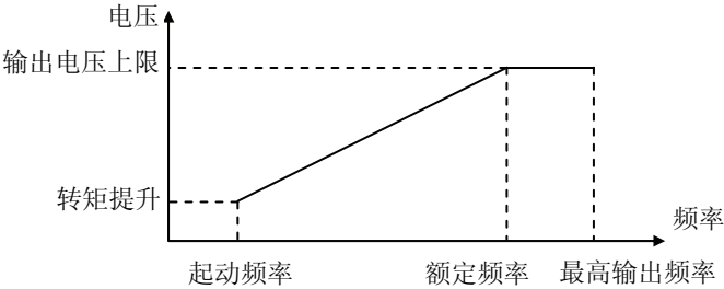
线性 V/F 曲线
