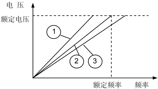
图 6-5 自动节能示意图
