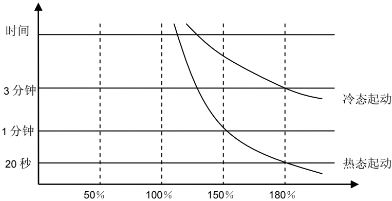
图 6-32 电子热保护
