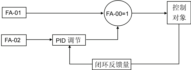
图 6-37 开环给定+PID 运行
