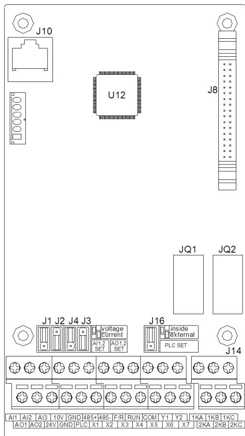
图 3-4 主板跳线插针示意图
