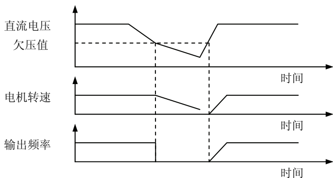
图 6-17 电恢复时频率从零起动
