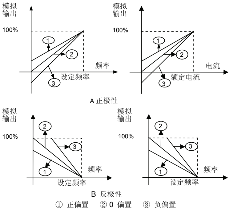
图 6-14 模拟输出信号
