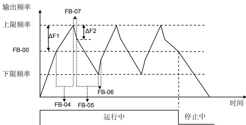
图 6-42 摆频范围和加减速
