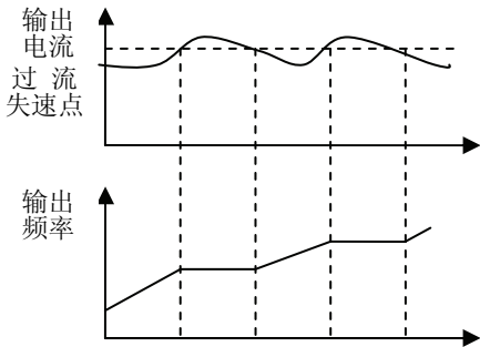
图 6-34 加速运行中过流失速控制
