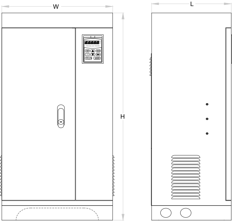
图 4：落地式安装（11KW-1000KW）
