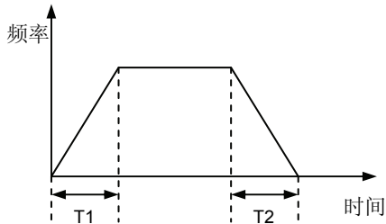
图 6-21 直线加减速
