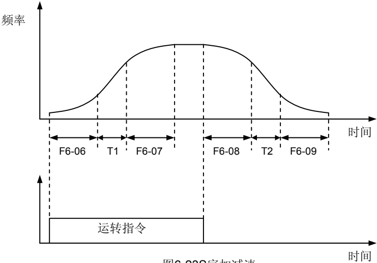
图6-23S字加减速
