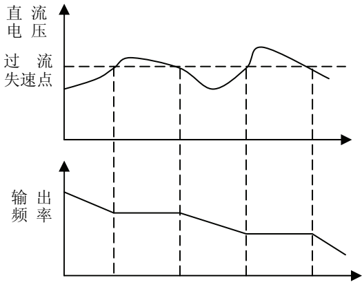
图 6-33 过压失速
