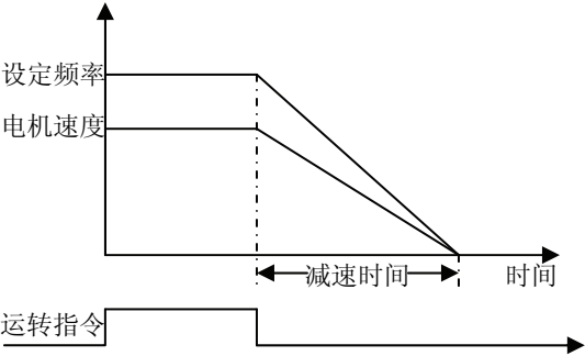
图 6-24 减速停车
