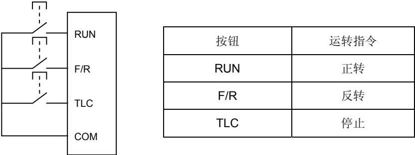
图 6-6 外控端子控制运行方式示意图
