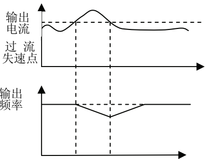
图 6-35 恒速运行中过流失速控制
