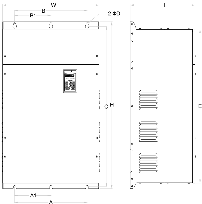
图 3：壁挂式安装（55KW-500KW）
