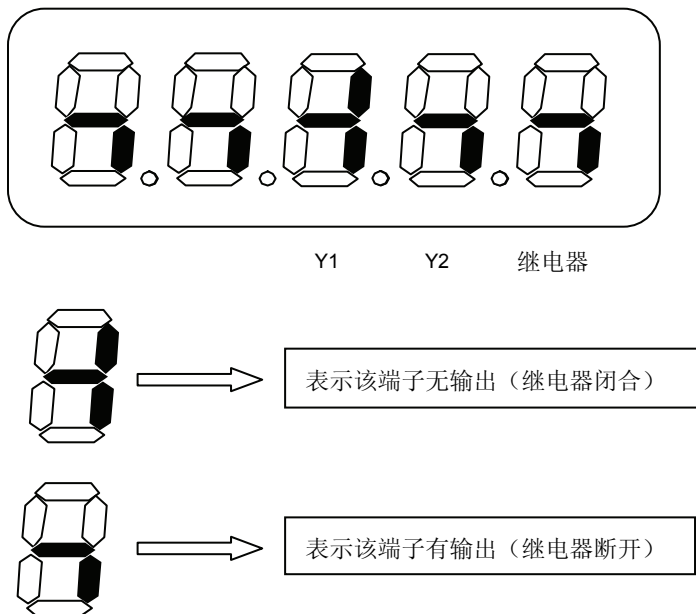
图 6-28 输出端子状态显示
