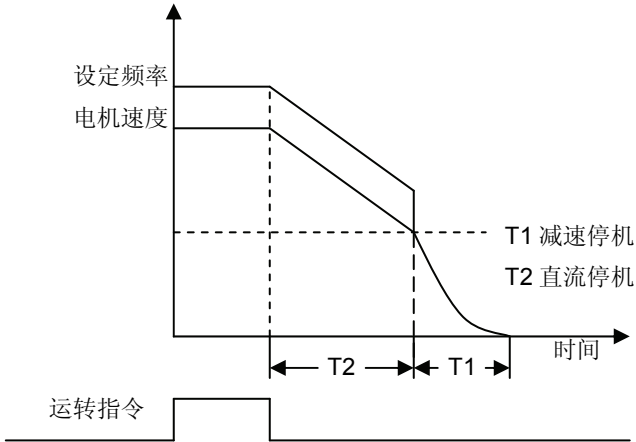
图 6-26 减速停车加直流制动
