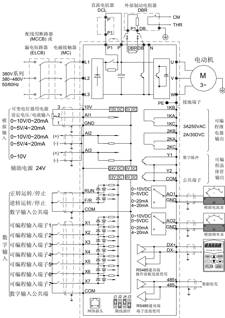
变频器接线图
