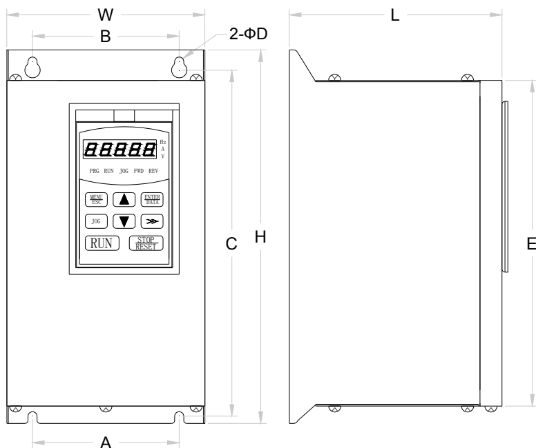
图 1：壁挂式安装（1.5KW-18.5KW）
