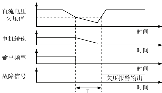
图 6-18 停电超时欠压保护 T > F6-02
