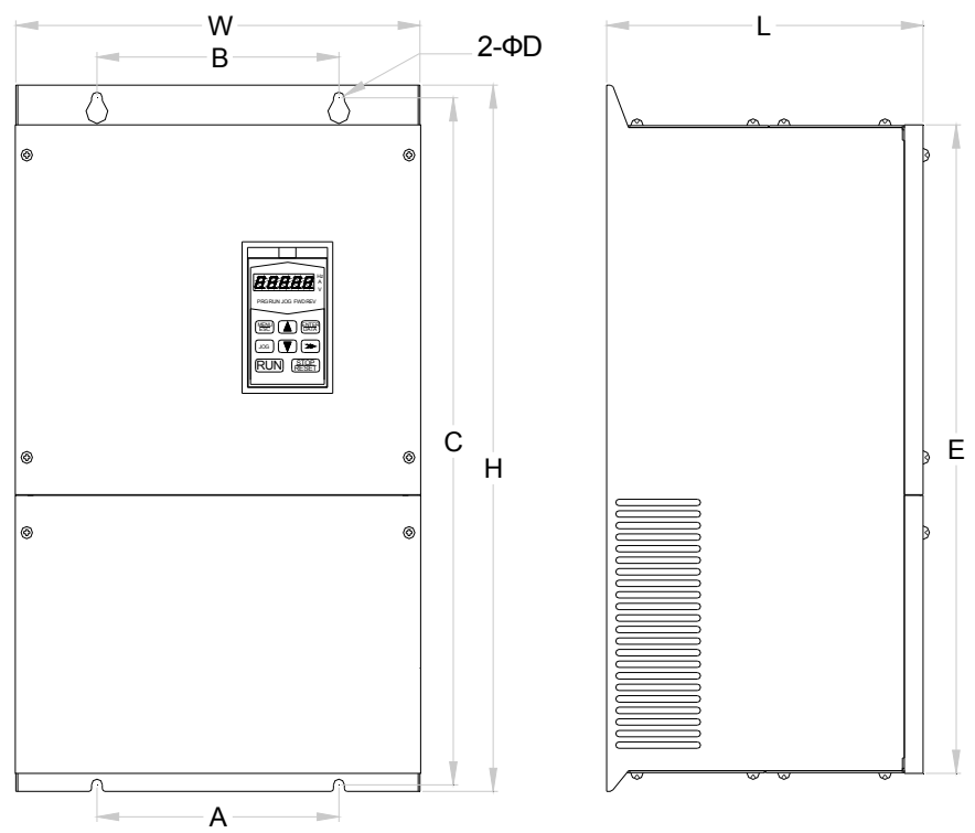
图 2：壁挂式安装（22KW-45KW）
