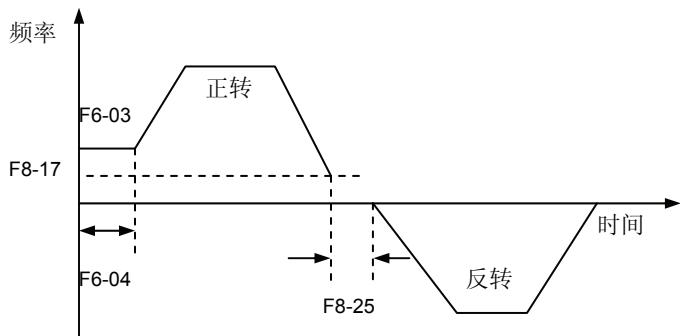
图 6-31 正反转死区时间
