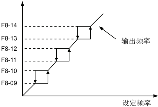
图 6-29 回避频率
