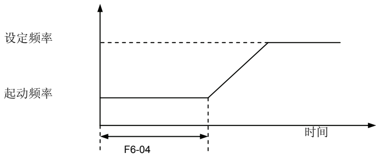
图 6-20 起动频率持续时间
