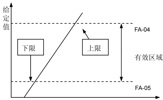
图 6-38 给定值限制
