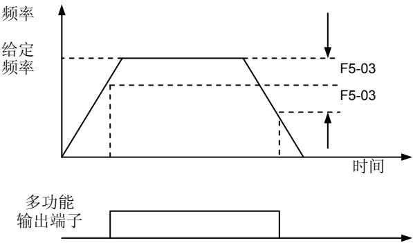
图 6-10 频率到达宽度
