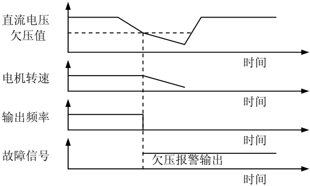
图 6-16 瞬停电时欠压保护
