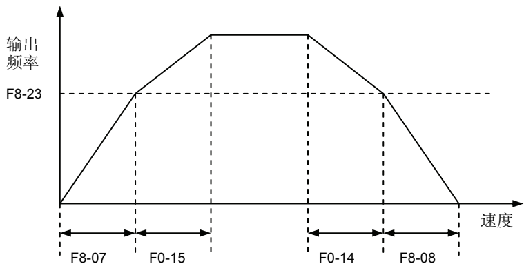
图 6-30 加减速切换频率
